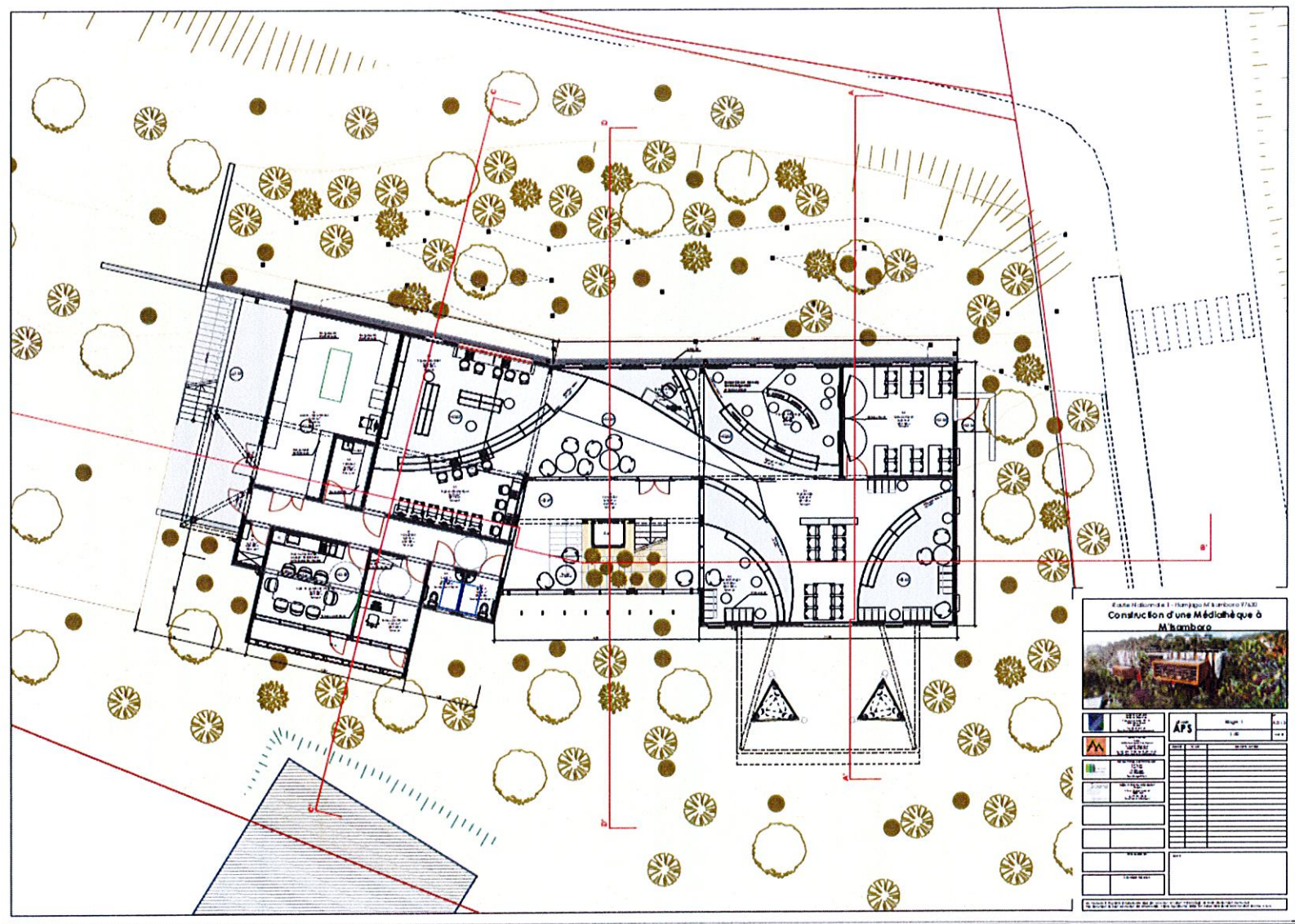
Figure 4: Plan du Rez-de-jardin - Extrait de l'APS
